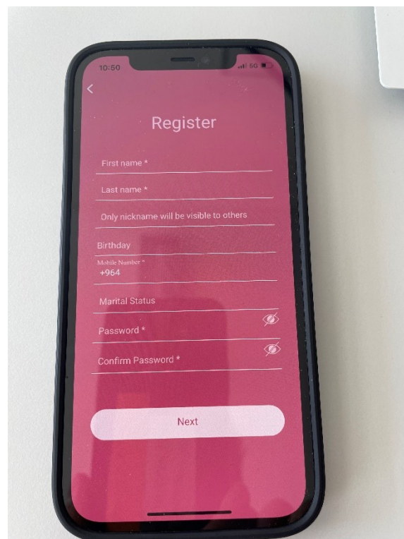
Abb. 15: Anmeldeseite.
